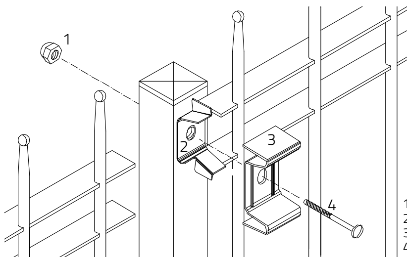
Bullone a testa tonda M8 x 55 e M8 x 65 con dado cieco. Finitura: inox.
